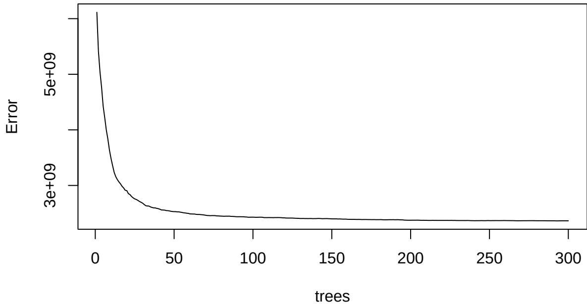
rf_model
